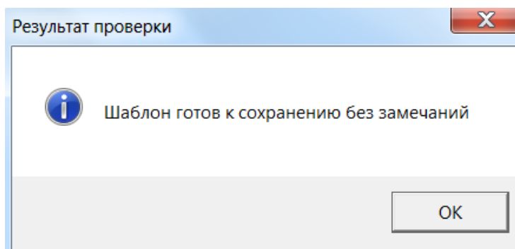
Рисунок 19 – Результат проверки
